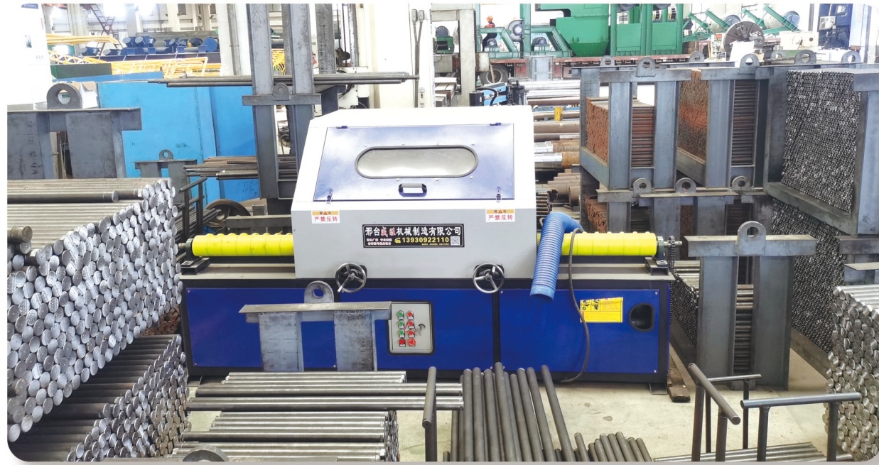
托辊清洗机
