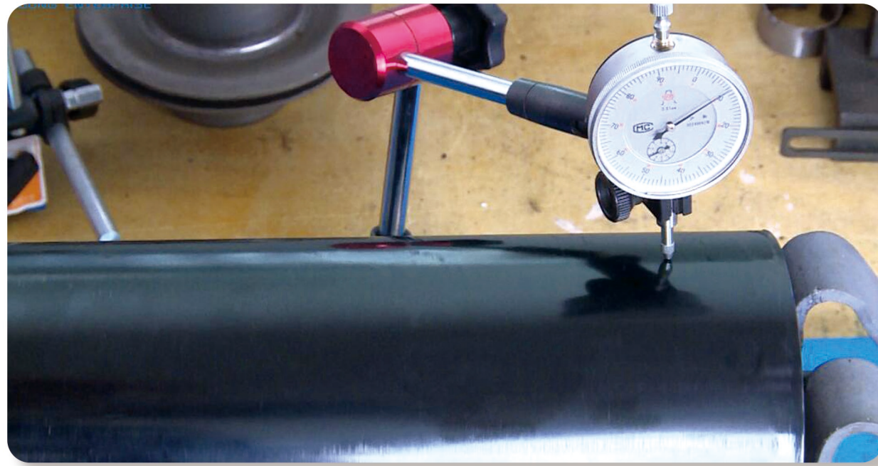
托辊径向跳动测试装置
